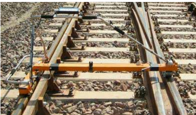
5. Przejazd przez krzyżownicę – nieciągłość toku szynowego
