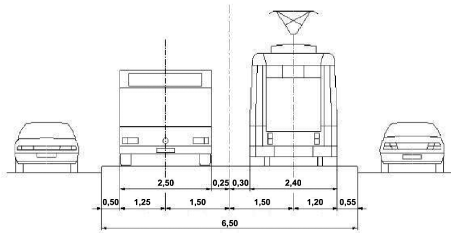
3. Zaproponowany przekrój pasa autobusowo-tramwajowego w Toruniu
