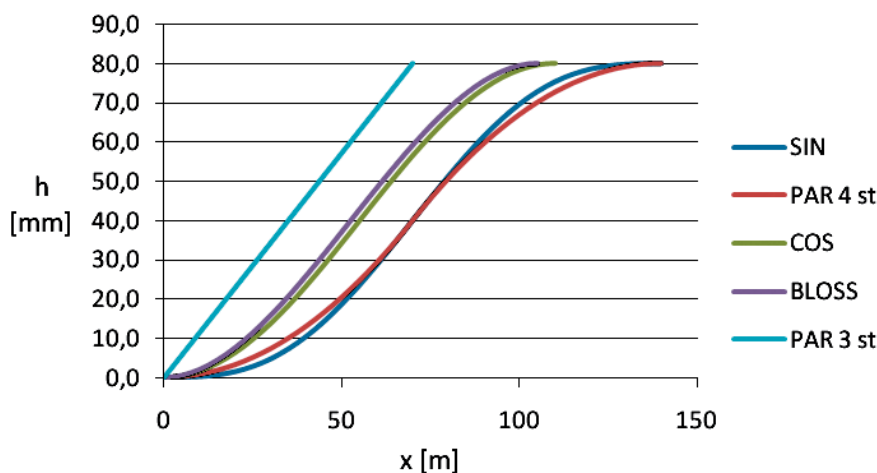
2. Kształtowanie się rzędnych rampy przechyłkowej na długości parabol trzeciego stopnia i gładkich krzywych przejściowych
