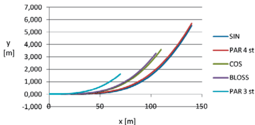
3. Kształtowanie się rzędnych poziomych na długości parabol trzeciego stopnia i gładkich krzywych przejściowych
