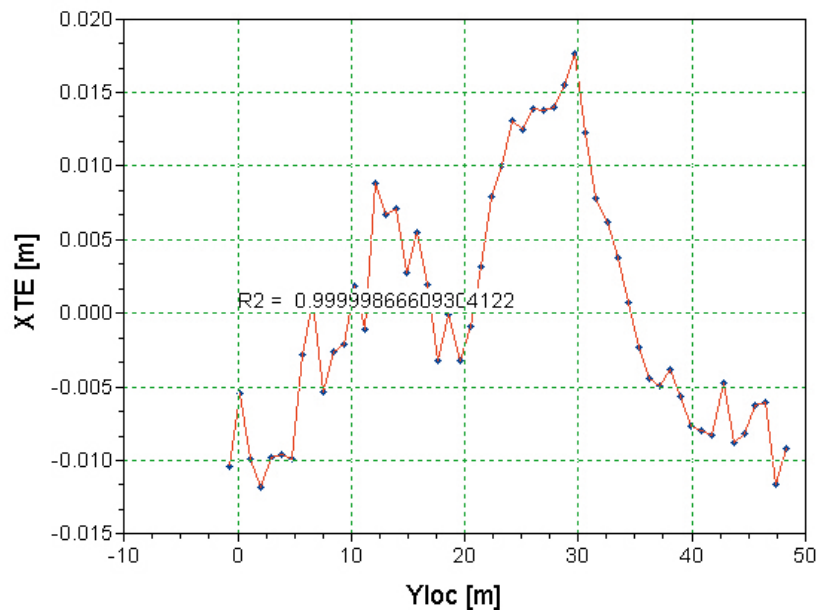
5. Określony ostatecznie sygnał XTE(Y_{loc}) reprezentujący wybrany odcinek prostej trasy (w skali skażonej)
