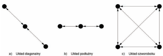
7. Wybrane warianty rozmieszczenia odbiorników GNSS względem osi podłużnej platformy w procesie wyznaczania osi toru
